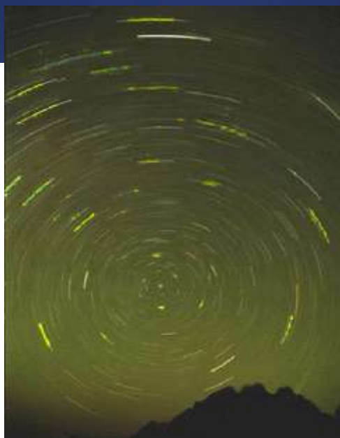
Polo Nord ripreso con tempi di esposizione fotografici di circa 1 ora
