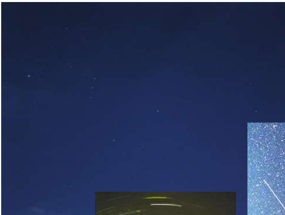
Costellazione di Orione (a sinistra) e di Andromeda con l'omonima nebulosa (in basso a destra)
