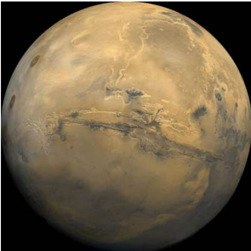
Marte (al centro Valles Marineris ed i vulcani di Tharsis in alto a sinistra della foto)
